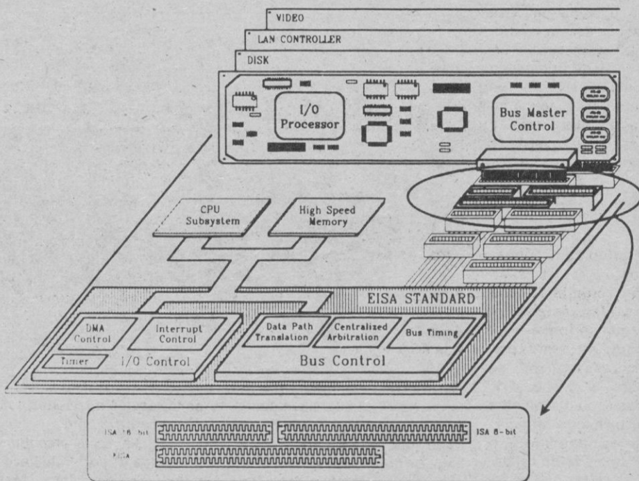
La nueva arquitectura EISA (Extended Industry Standard Architecture) compete con la Micro Channel de IBM y la de Apple para ganar la carrera de los PC futuros. —(Foto Efe)
