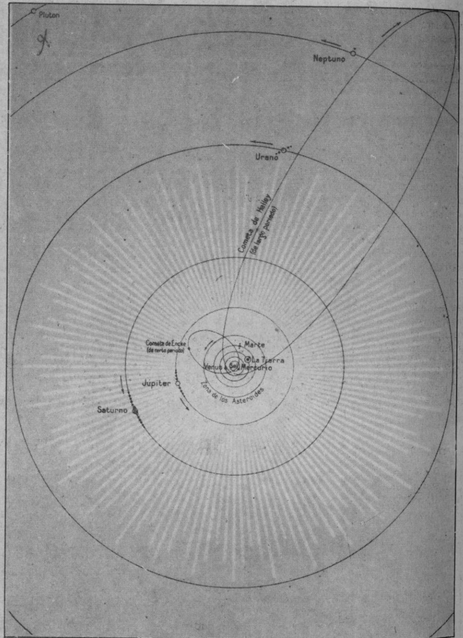
Los cometas proceden de la nube de Oort, más allá de los planetas, atraviesan las órbitas de éstos y giran en sentido contrario
