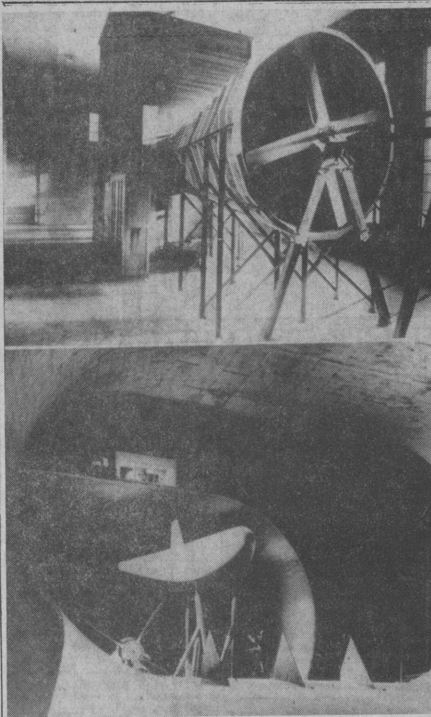
Langley (Hampton, EE. UU.).—Arriba, el primer túnel aerodinámico de mil novecientos diecisiete, del Centro de Investigaciones de Langley, Hampton. Abajo, el túnel del mismo Centro empleado actualmente para los ensayos de la N. A. S. A. (Administración de Aeronáutica y del Espacio). El Centro acaba de cumplir cincuenta años. Creado en mil novecientos diecisiete para el estudio del carenaje de motores de avión, luego de dirigibles, posteriormente de aviones modernos y supersónicos, actualmente se dedica al estudio de satélites.—(Foto Europa Press)
