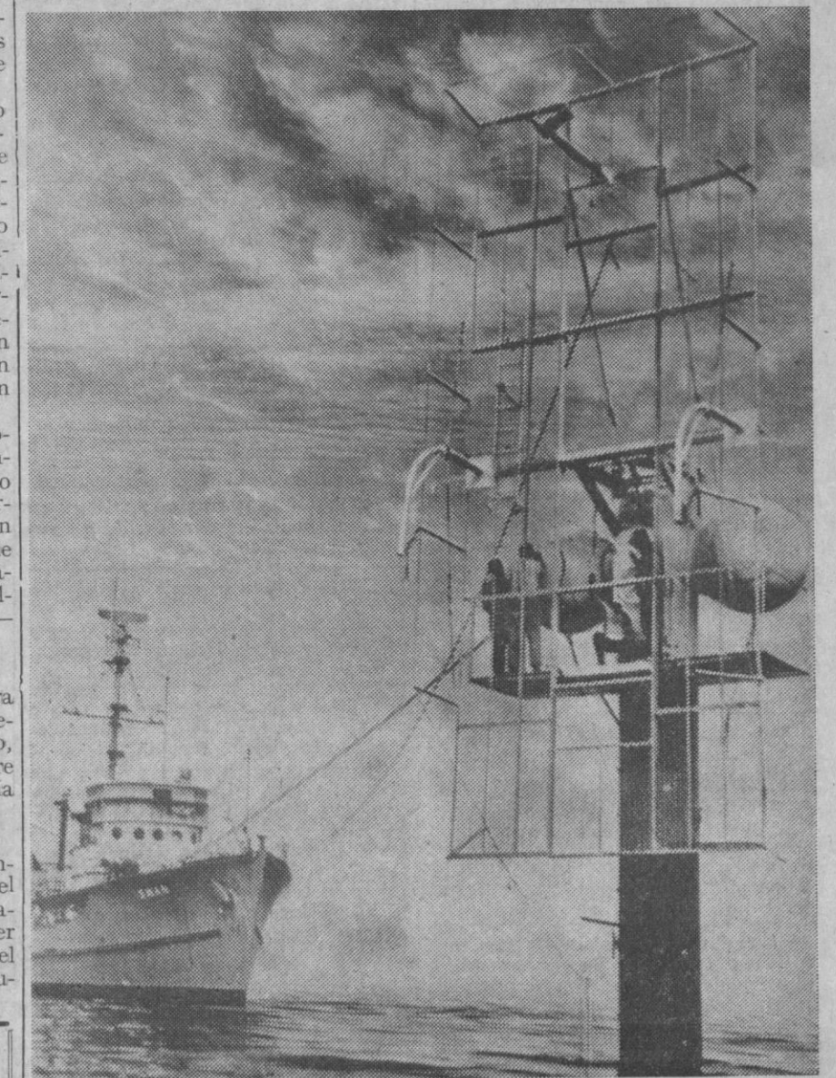
En aguas de California.—Desde la plataforma marítima (derecha) se prueba un nuevo «sonar» que recoge los sonidos de todo objeto que navegue por encima o por debajo del agua, tan sensible que puede distinguir unos de otros. A través del barco de investigaciones «Swan» (izquierda) la información se extiende en tres dimensiones sobre la pantalla situada en tierra firme, a unos treinta y cinco kilómetros de distancia.—(Foto Europa Press)
