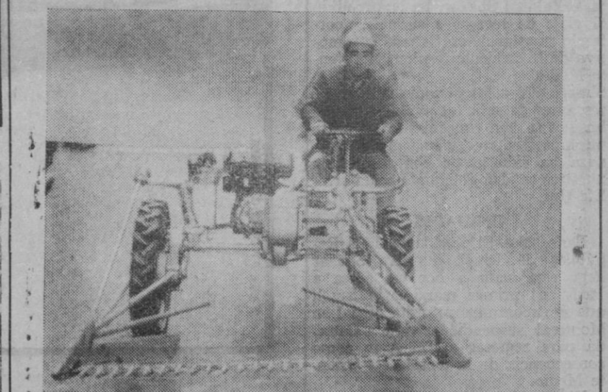
La máquina que siega hierba y se adapta a siega de mieses con atador
