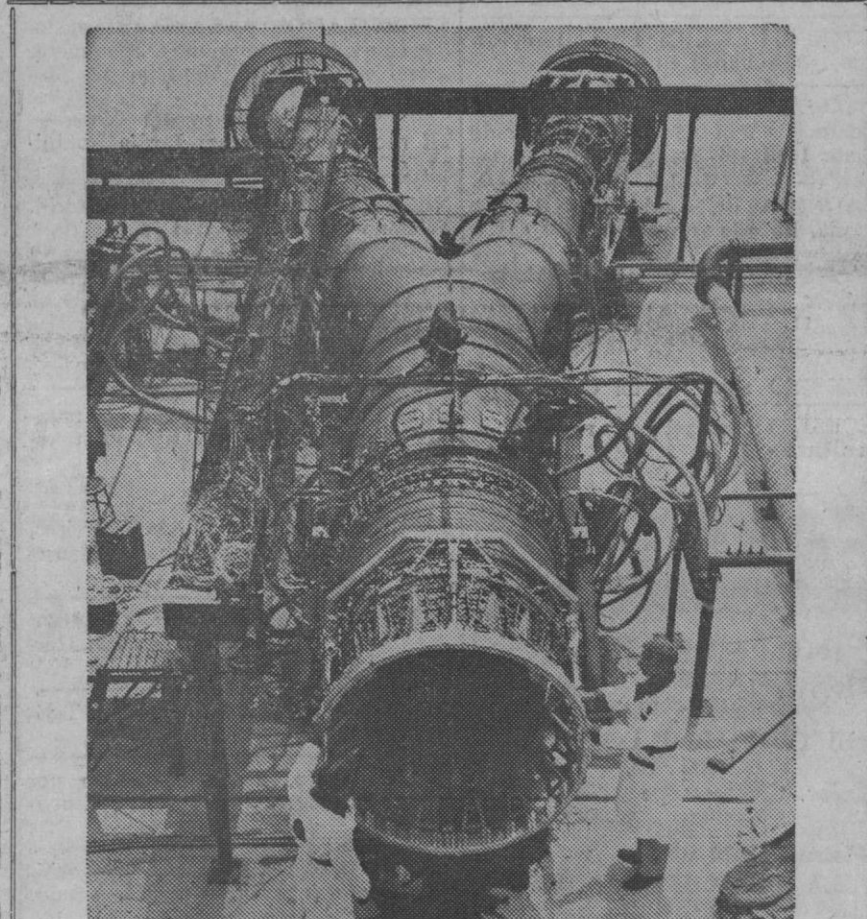
Este singular dispositivo de investigación en forma de horquilla es utilizado para someter a prueba componentes de motores para los aviones norteamericanos supersónicos de transporte (SST) del futuro. En cada uno de los dos extremos posteriores del aparato hay montado un motor jet corriente para generar en la cámara que aparece en primer plano el alto volumen de corriente de aire y las altas temperaturas necesarios para duplicar el proceso de combustión de los futuros motores
