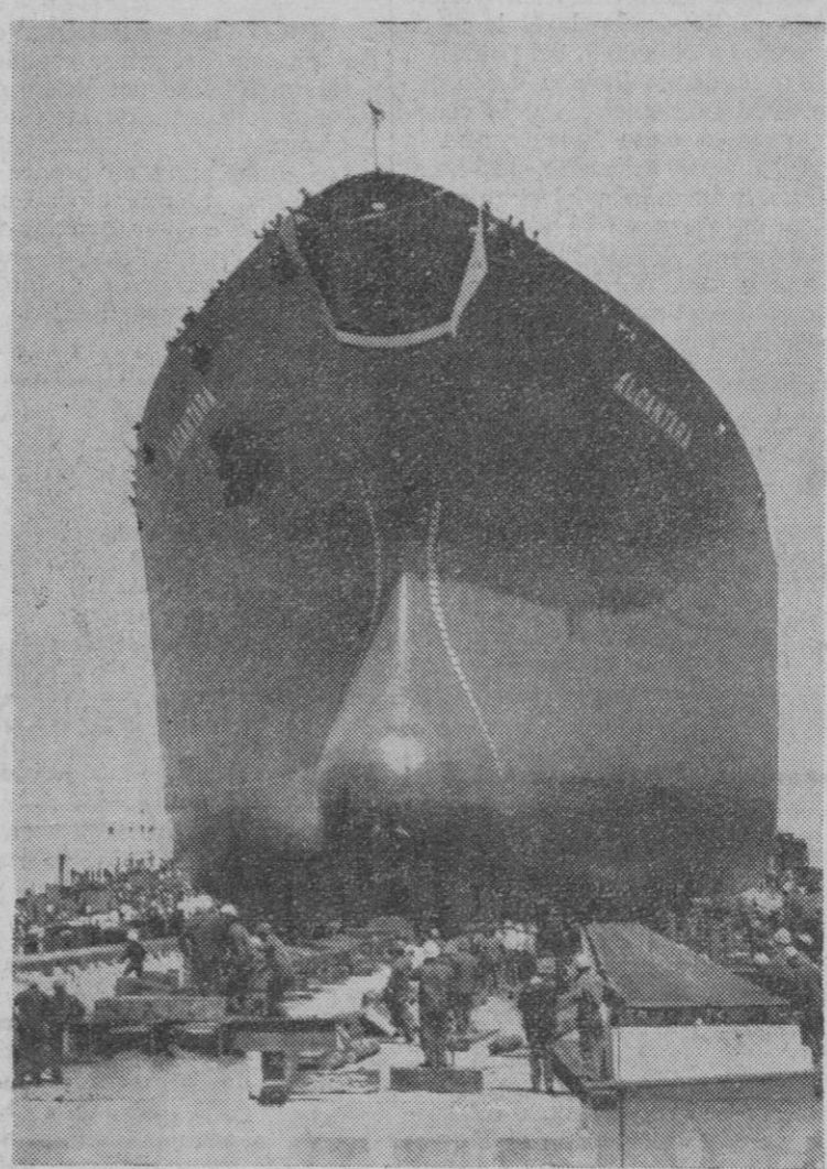
En la factoría de Astilleros de Cádiz ha sido botado el gigantesco petroquímico "Alcántara", de sesenta y seis mil toneladas de peso muerto. Ha sido construido por encargo de la refinería de petróleo de Escombreras, y puede alcanzar una velocidad de diecisiete nudos con una autonomía de doce mil millas. Actuó de madrina en la botadura la esposa del ministro de Industria, doña María Angeles Velasco de López Bravo, estando su esposo presente en la ceremonia. Vemos en la foto un momento de la botadura del buque. (Foto Fiel)
