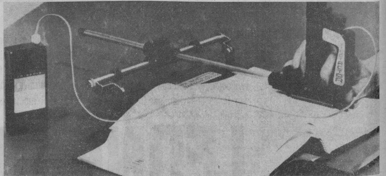
Dagones (Ohio, EE. UU.).—Este es el «Visotactor», instrumento de lectura para ciegos. Traslada imágenes escritas a vibraciones, mediante pulsaciones. Tiene el tamaño de una pistola pequeña. Puede «leer» desde una obra de Shakespeare a la etiqueta de un bote de conservas. Fabricado en unos laboratorios de esta ciudad, consiste en células fotográficas y vibradores. Metiendo los dedos de la mano derecha dentro de cuatro agujeros y moviendo el aparato a través de la página, el invidente recibe vibraciones equivalentes para él a letras.—(Foto Europa Press)
