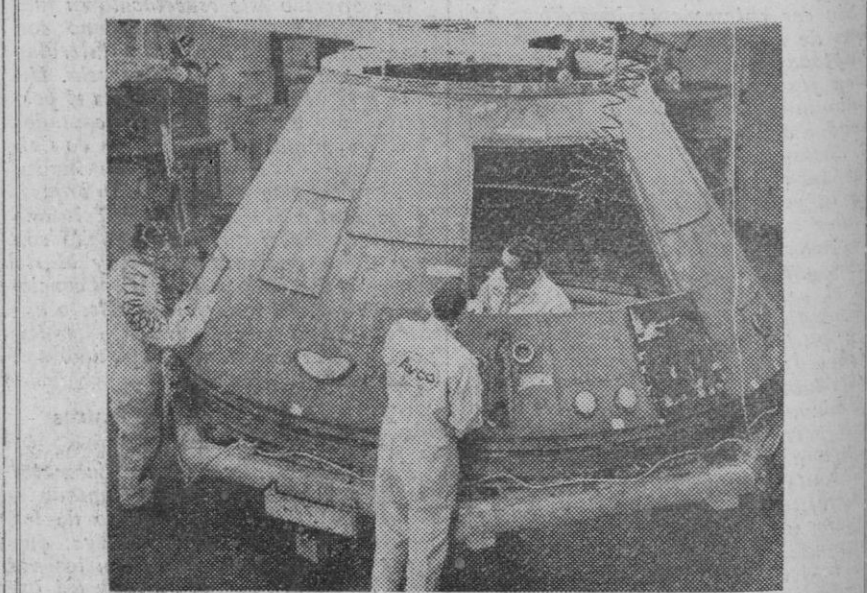
Tres expertos de la fábrica "AVCO", de Lowell (Massachusetts), terminan de armar el blindaje térmico para la astronave Apolo. El blindaje se compone de trescientas cincuenta mil celdas a manera de panel llenas de un material aislador y protegerá a los tres astronautas de la tripulación del efecto de las atmósferas sumamente altas generadas por la fricción atmosférica durante el trayecto de regreso de la nave a la Tierra después de su vuelo de exploración
