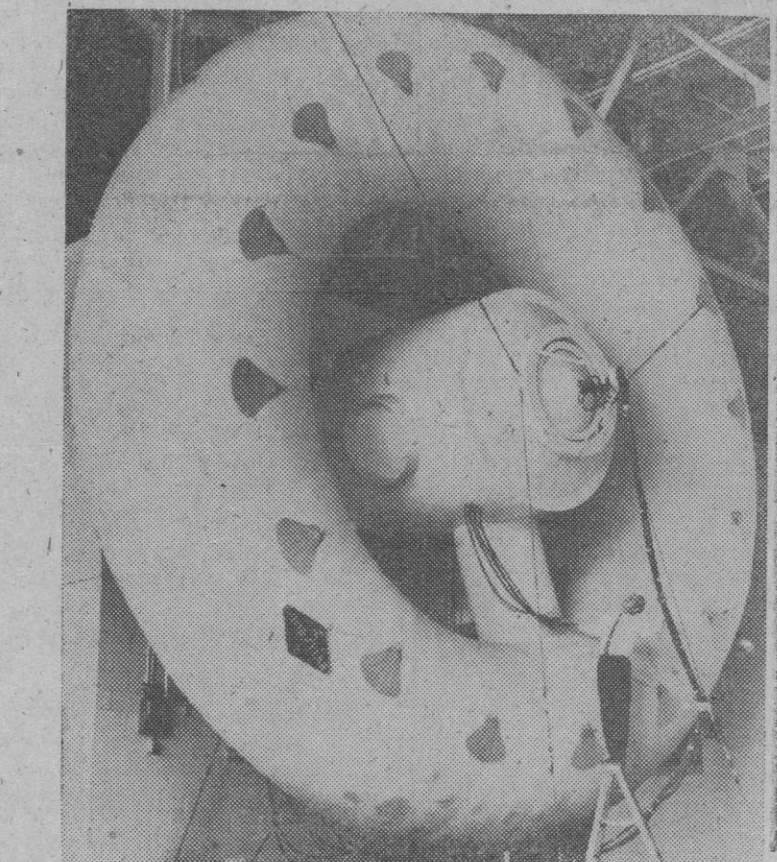
En el Centro de Investigación Lewis que en Cleveland (Ohio, Estados Unidos) tiene instalado la NASA, un ingeniero inspecciona este modelo de tamaño natural de una estación espacial extensible. El ingenio tiene una altura de tres pisos y la forma de una rosquilla.
