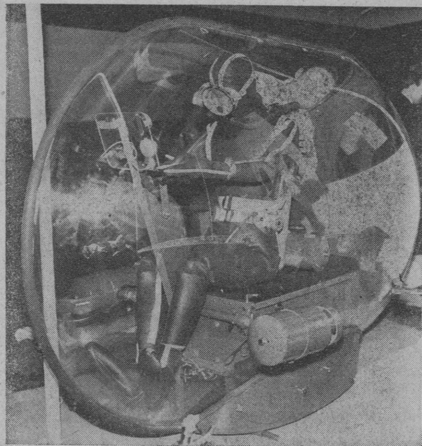
El capitán de corbeta H. H. B. Oswell, inglés, da los últimos toques al submarino de plástico por él construido, cuya tripulación se compondrá de tres hombres, y que se cree es el primero en su clase en el mundo. El submarino ha sido proyectado para facilitar el trabajo de los buzos que efectúan prolongadas tareas de observación e inspección, ya que su perfil aerodinámico proporciona amplia visión en derredor, a la vez que protección contra los riesgos submarinos
