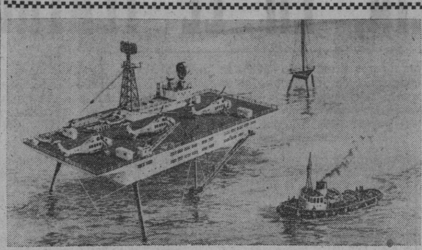
Nuevo tipo de plataforma marina que no flota ni se apoya en el fondo del mar, y tiene muchas aplicaciones en trabajos de aguas de gran profundidad que requieren una plataforma. La plataforma sobresale unos quince metros de la superficie y está sostenida por unos soportes que se apoyan en un tanque de flotabilidad, el cual está a su vez fondeado con cable en el lecho del mar. Entre las posibles aplicaciones de la plataforma se cuentan: exploración petrolera submarina, reconocimientos geológicos, terminales para buques, estaciones de radar y de navegación y para aterrizajes de helicópteros, como muestra esta impresión de artista
