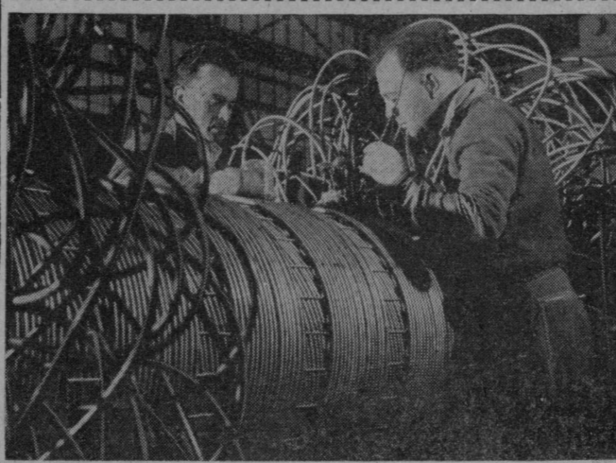
Obreros especializados desenredan una maraña de tuberías para montarlas en forma circular en un cambiador térmico que se halla en construcción en los talleres de una firma británica de ingeniería. Este cambiador, llamado cambiador "frío", es un enfriador de evaporación de nitrógeno para una planta de obtención de oxígeno líquido. En el enfriador, el aire comprimido pasa a través de tubos. El frío se transfiere al aire desde una mezcla de nitrógeno residual y agua que circula en torno de los tubos en contracorriente. La planta de oxígeno líquido producirá mil seiscientos metros cúbicos de oxígeno por hora para un campo de pruebas de motores de cohele
