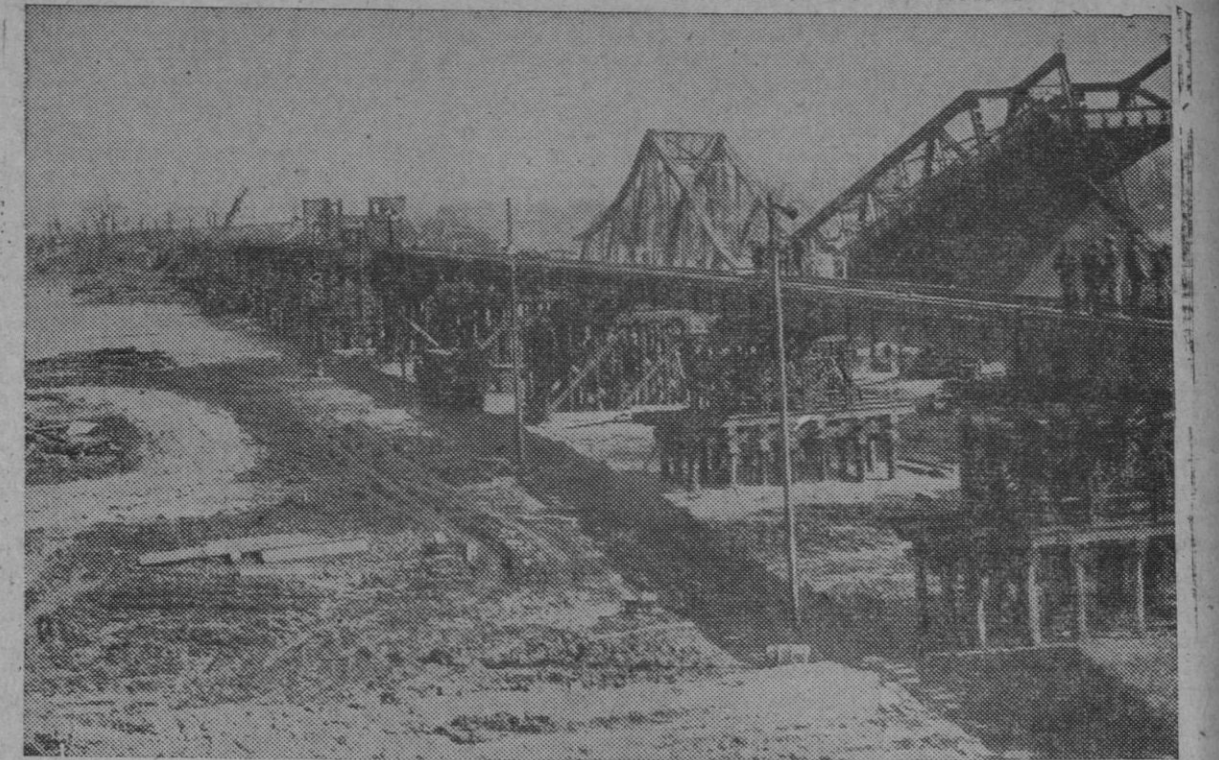
Un puente Bradley, construido por los ingenieros británicos en diez días. Este puente ha sustituido a uno volado por los alemanes en el Rhin
