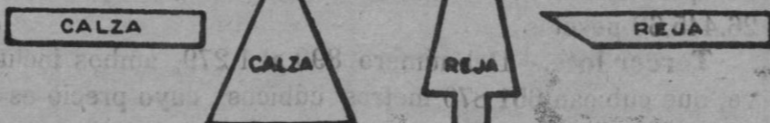
RECORTES Y PLETINAS PARA FABRICACION DE HERRADURAS
