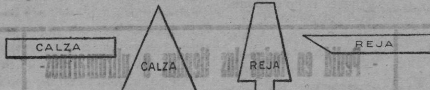
RECORTES Y PLETINAS PARA FABRICACIÓN DE HERRADURAS.
