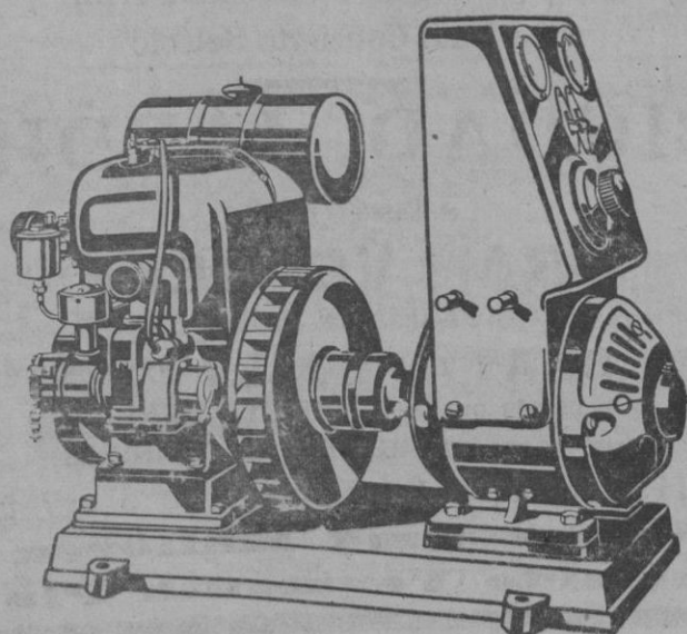
Grupo Electrogeno
