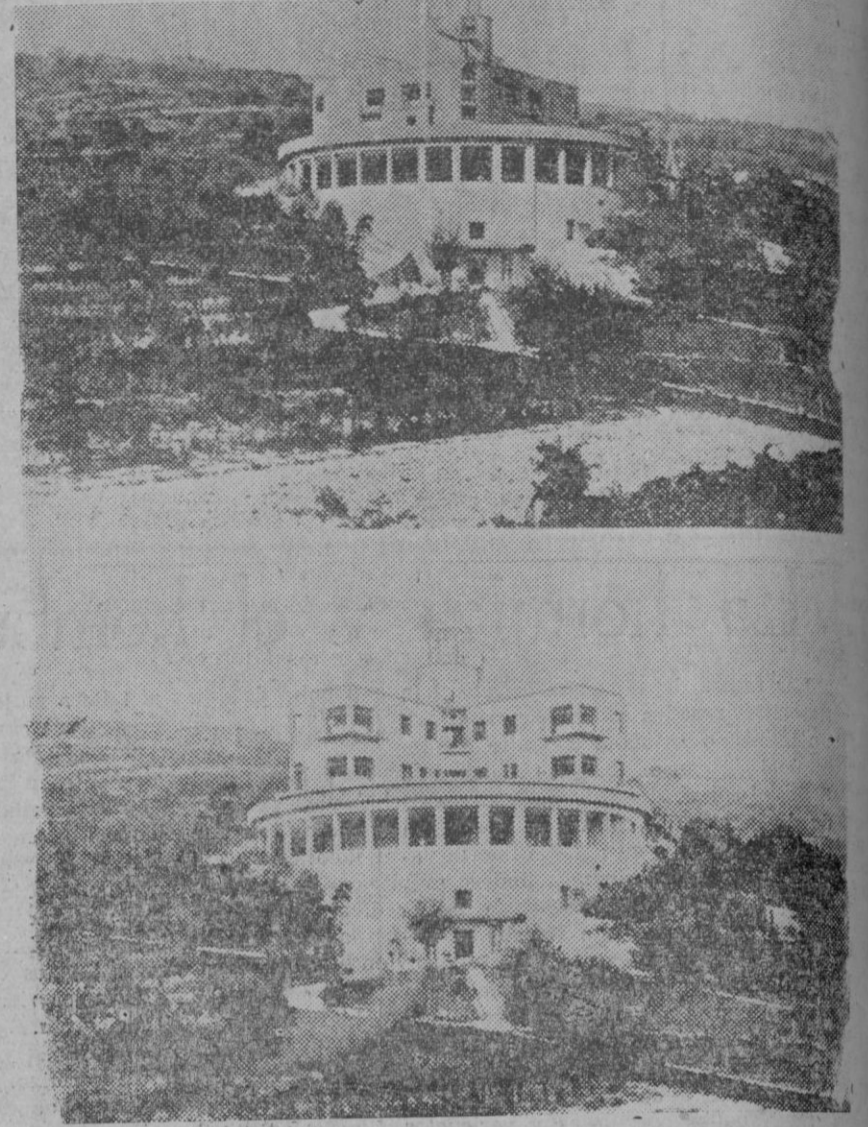
UNA CASA QUE SIGUE EL MOVIMIENTO DEL SOL. — El ingeniero italiano Angelo Invernizzi se ha construido una casa cuya fachada sigue durante todo el día el movimiento del sol. un potente motor hace girar el segundo piso de la casa. Dos aspectos de la casa girasole cerca de Veron. La casa fotografiada desde el mismo punto por la mañana y por la tarde. (Express Foto).
