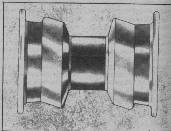
La nueva llanta asimétrica Pirelli Goodyear difiere poco de las llantas standard y puede ser montada con todos los radiales sin cámara, en pulgadas, empleando equipos de montaje y métodos standard. La llanta Goodyear Pirelli es ya equipo standard del Fiat Abarth 130 TC.
