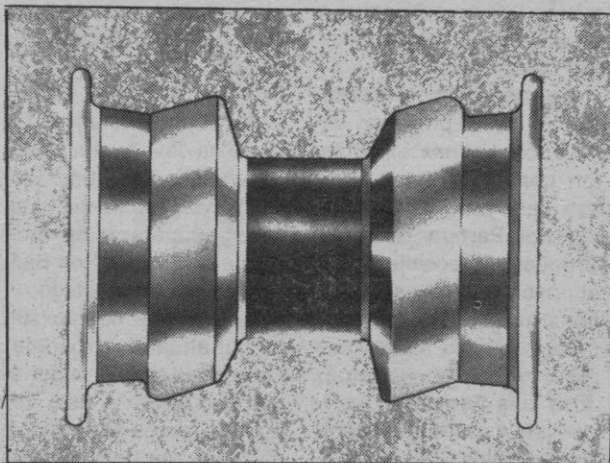
Imagen de la nueva llanta asimétrica Pirelli Goodyear, mostrando la llanta en una de sus modalidades de operatividad. Con esta nueva llanta, el descalzamiento del talón sucede a una presión entre 0 y 0,34 bar, según la dureza de condiciones. Los automovilistas pueden mantener un control más positivo y de movilidad del vehículo con la llanta Goodyear Pirelli después de una pérdida de aire.
