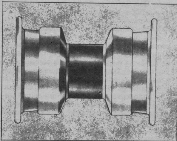
Imagen de una llanta standard para coche, mostrando una única guía de retención de los talones del neumático, situada simétricamente a cada lado de la llanta. En una severa maniobra en curva de un coche con neumáticos montados en llantas standard estos se destalonan y caen en el canal de la llanta aproximadamente a 1 bar. Esto puede representar la pérdida del control del vehículo.
