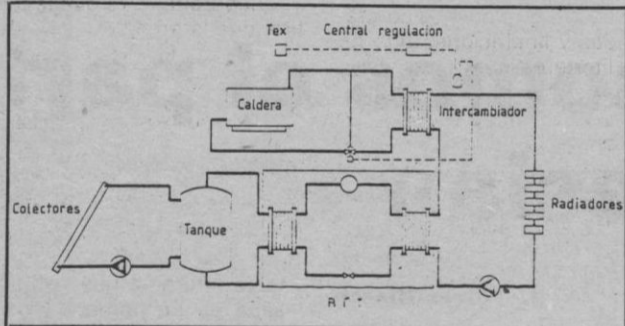
El sistema, que combina las antiguas calderas de fuel con las modernas por energía solar, son sumamente sencillas.
