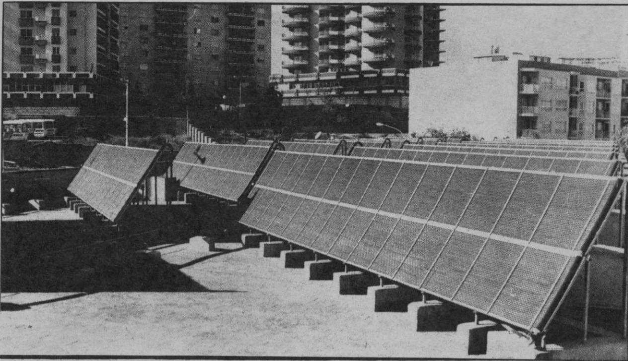
200 metros de colectores de caucho captan la energía solar que es almacenada en un tanque de agua enterrado y perfectamente aislado.
