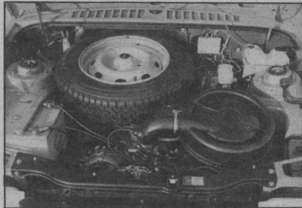
El motor queda bastante desahogado en el vano motor, sobre todo cuando se quita la rueda. (Foto Vives)
