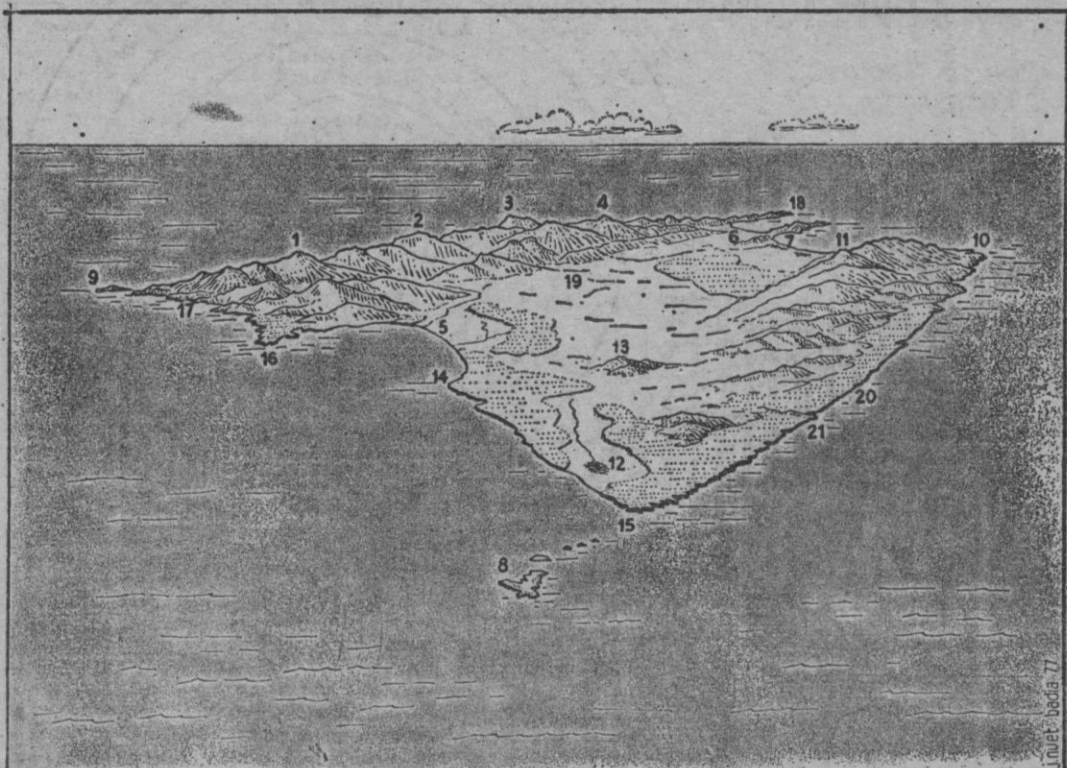
Diagrama morfológico de la isla de Mallorca, según dibujo de G. Colom, donde se destaca la Serra de Tramontana.
