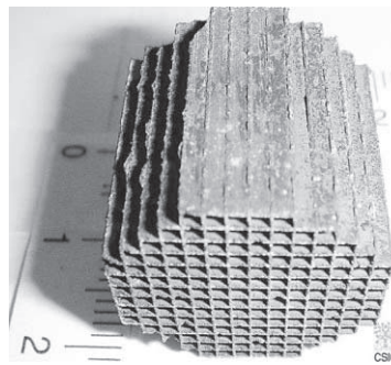
Imagen del catalizador desarrollado por los investigadores españoles
