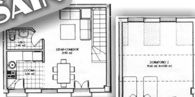
PLANTA ALTA
