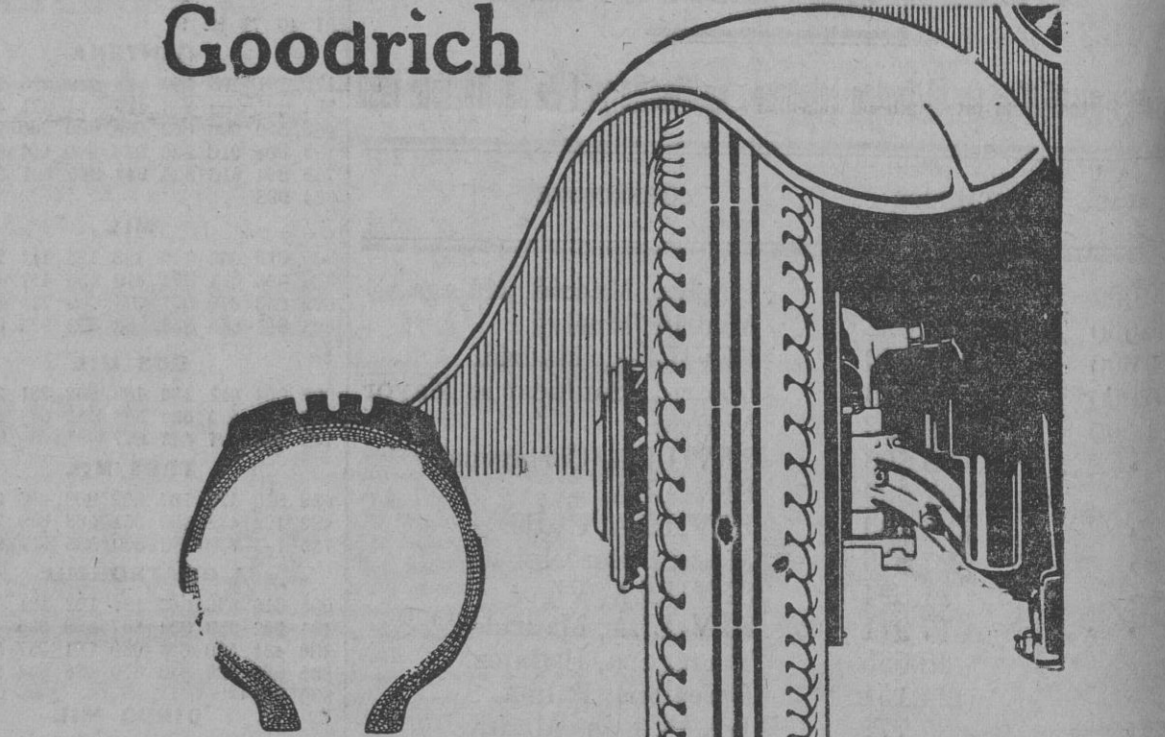
A la derecha el dibujo de la famosa banda de rodamiento Goodrich. El desgaste es muy reducido gracias a la composición de su goma y a la taja que lleva en el centro de la banda
