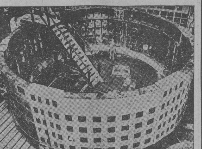
La exportación alemana continúa, a despecho de la guerra. En los talleres Siemens se están terminando cuatro dinamos hidroeléctricas, del mayor tamaño construido hasta ahora en Europa, con destino a Corea y Manchukuo. (Foto Weiblich.)
