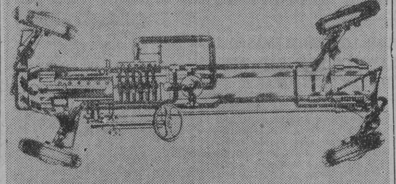
Esquema del automóvil de tracción hidráulica del inventor español, don José Tous Forrellad. — (Foto Cifra)
