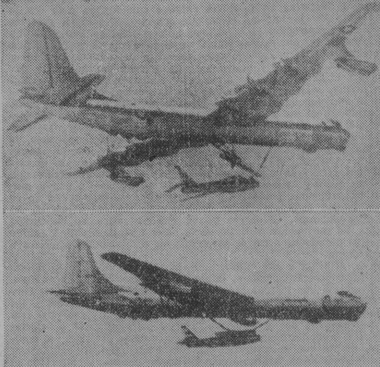
UN PORTAAVIONES VOLANTE. — Las fuerzas del aire norteamericana, nos efectuaron el pasado día 25 del actual, unas pruebas con un bombardero «B-36», especialmente acondicionado como portaaviones. El aparato puede llevar suspendido otro avión — en la prueba fué un «F-84F» de reacción — que en un momento dado puede soltarse para volver otra vez al bombardero, en pleno vuelo. El «portaaviones volante» es el bombardero más grande del mundo, y lleva seis motores de explosión y cuatro de reacción. Su velocidad media es de 435 millas por hora, pudiendo llegar hasta las 600 millas, siendo su radio de unas 10.000 millas. En las fotos pueden verse dos fases diferentes del «despegue» y «amarre» del pequeño avión «F-84F». — (Foto Associated Press)
