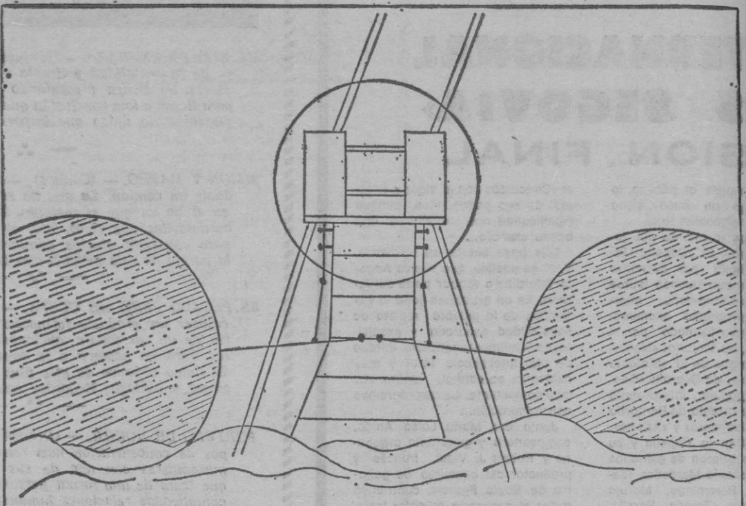
El movimiento de las olas es transformado, mediante los bidones flotantes, en el bombeo de agua para su elevación.
