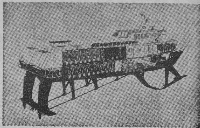
Año 1968: Hidroala «EXPRESSAN» serie Supramar PT-150 DC construido en Mandal para realizar la travesía entre Gothenburg (Suecia) y Frederikshavn (Dinamarca) a través de los estrechos de Cattgat y Skagen Rak que unen el Mar del Norte con el Mar Báltico.
