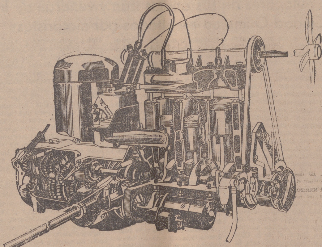
He aquí el detalle del magnífico motor de la DKW en su versión de gasolina, que tanto prestigio ha proporcionado a los vehículos lanzados por IMOSA.
