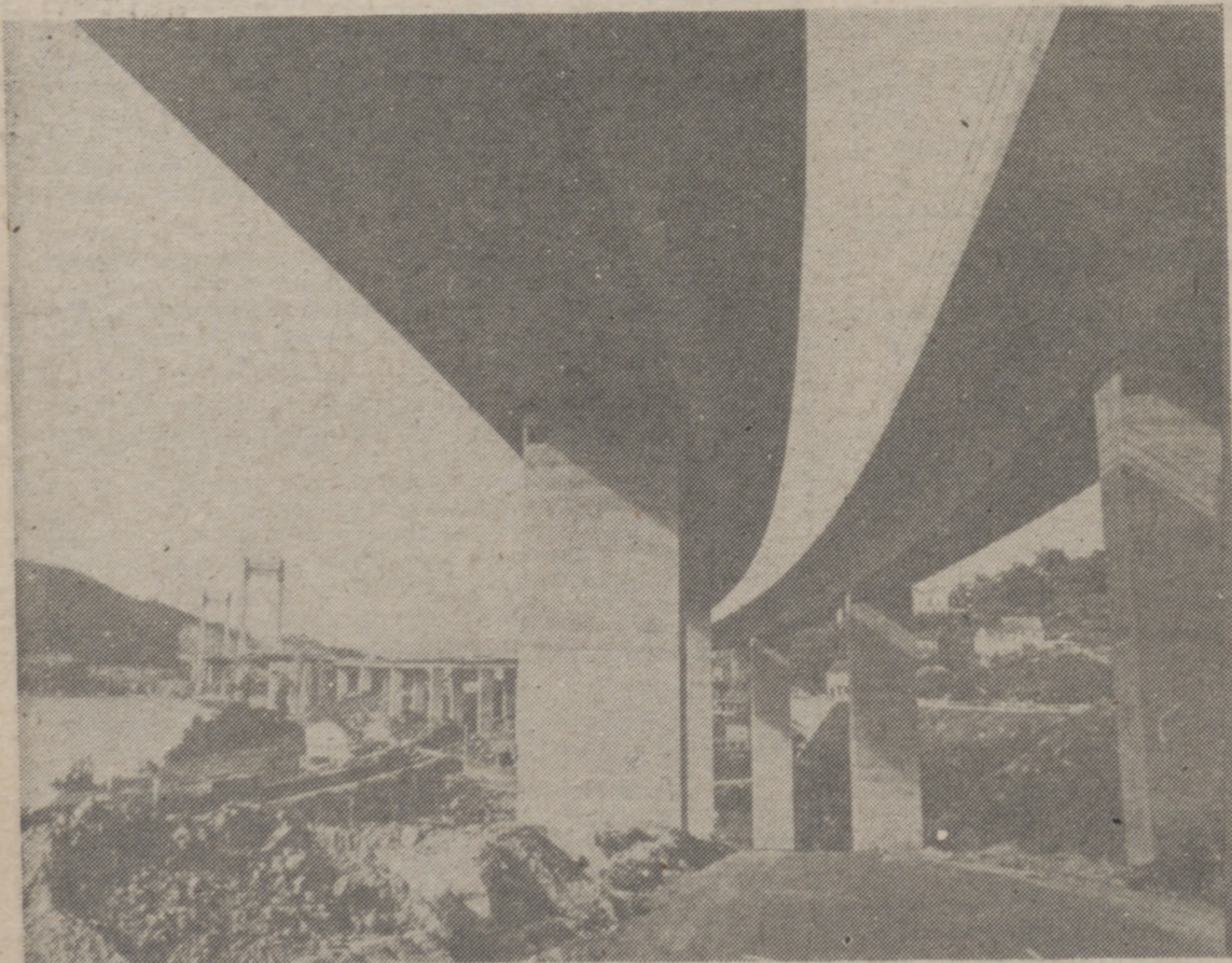
VIGO.—A finales de este verano quedará inaugurado y abierto al tráfico este soberbio puente de Rande que, como parte de la autopista del Atlántico, une Vigo con la península del Morrazo. El puente con vano central y laterales de hierro, tiene una longitud de 1.600 metros, 23 metros de anchura (cuatro carriles para cada dirección) y un coste total de 2.100 millones de pesetas. La pila central con sus 128 metros de altura, bate el récord de España en este tipo de construcciones. (El anterior estaba en 98,5).—(Foto Cifra Gráfica.)
