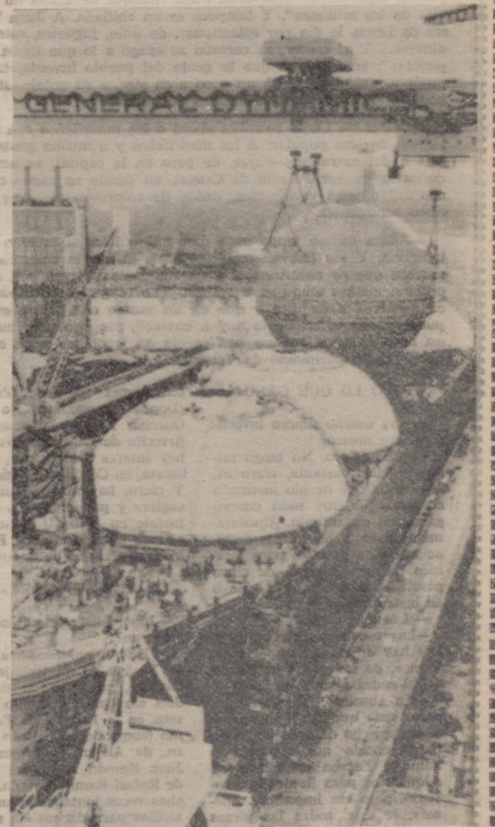
QUINCY (Mass.).—En los astilleros de la General Dynamics se ha construido un barco de 936 pies de eslora, donde albergará doce tanques contenedores para transportar gas natural licuado. De este modo, el barco podrá llevar 125.000 metros cúbicos de dicho gas a una temperatura no inferior de 265 grados. (Foto Cifra Gráfica-Upi.)
