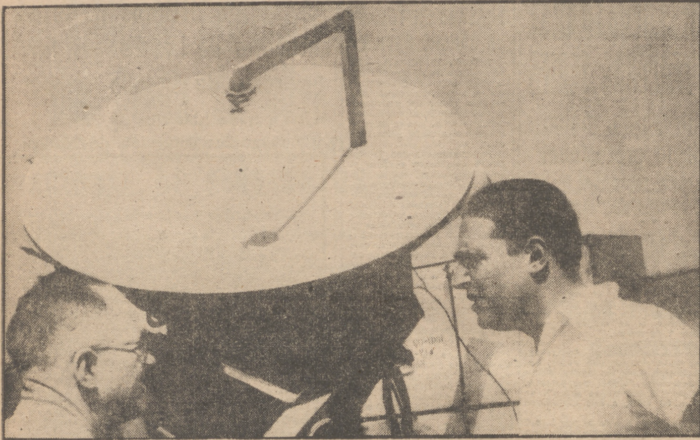
Este radiómetro de diez milímetros es una de las piezas del equipo que ha utilizado la expedición del Laboratorio de Investigaciones de la Marina norteamericana y del Observatorio de gran altura de Boulder (Colorado), en Khartum (Sudán angloegipcio) para presenciar el eclipse de Sol de ayer, lunes. Alrededor de cien científicos de numerosos países llegaron a Khartum. (Foto Cifra.)
