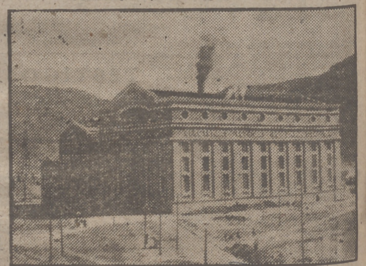
Fachada posterior y estructura de transformación de la central
