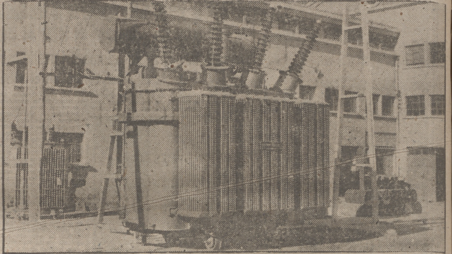
Transformador de 12.000 kv., tensión 132.000 v.
