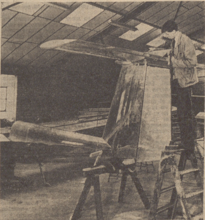
Vista de cerca de la parte trasera del fuselaje del T-53 mostrando el alto plano horizontal de cola. Los veleros están diseñados para un desmontaje rápido de los principales componentes, y no se necesita una escalera para desmontar el plano horizontal, como podría sugerir esta fotografía
