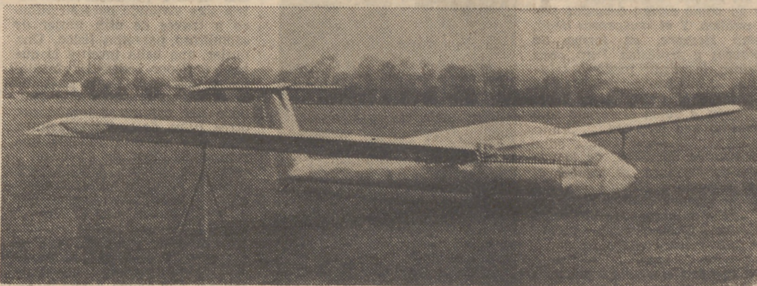
El T-53 en el aeródromo de pruebas de los fabricantes en Kirby-Moorside. Con claridad se aprecia la gran cubierta de la cabina (que cubre a ambos ocupantes), la rueda sencilla principal y la pequeña rueda del morro, así como el ala de elevado alargamiento y el plano horizontal de cola montado en la parte superior del estabilizador vertical
