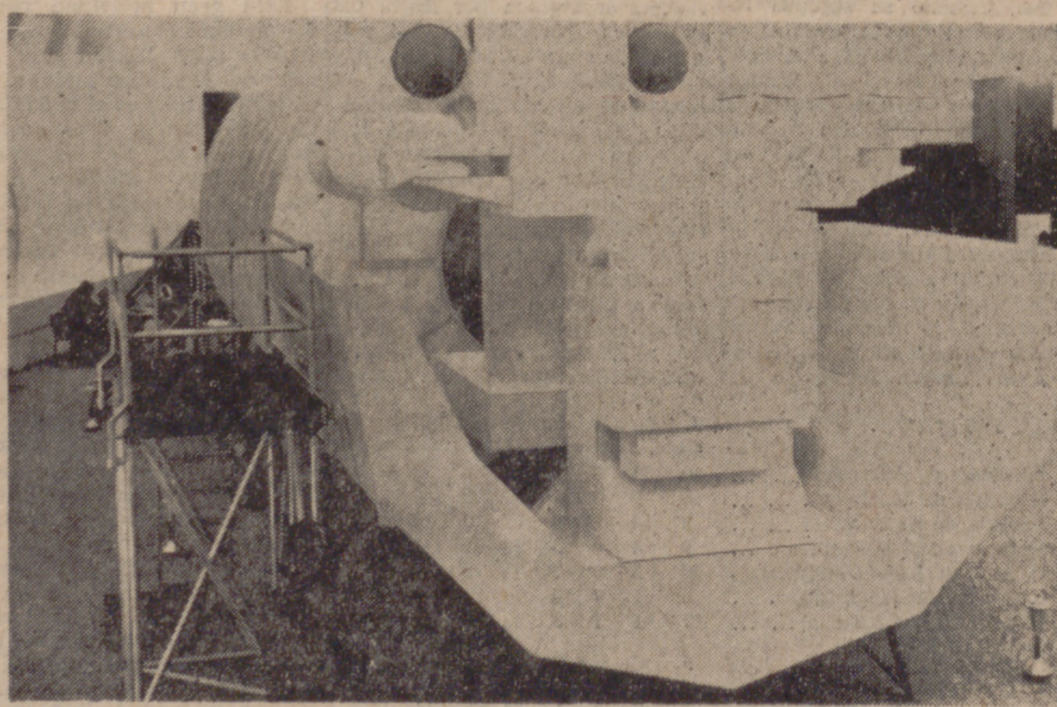
BREMEN. (DaD).—En las dependencias del aeropuerto de Bremen acaba de ser presentado a la Prensa y a científicos de todo el mundo el modelo, en tamaño original, del laboratorio espacial diseñado y proyectado por la Organización Espacial Europea ERNO. En la realización de este proyecto conjunto de nueve países europeos se han invertido hasta ahora más de mil millones de marcos. En el interior del mismo irá instalado un laboratorio de ocho metros de longitud en el que podrán trabajar cuatro científicos. El primer lanzamiento de este laboratorio espacial europeo tendrá lugar en 1980.
