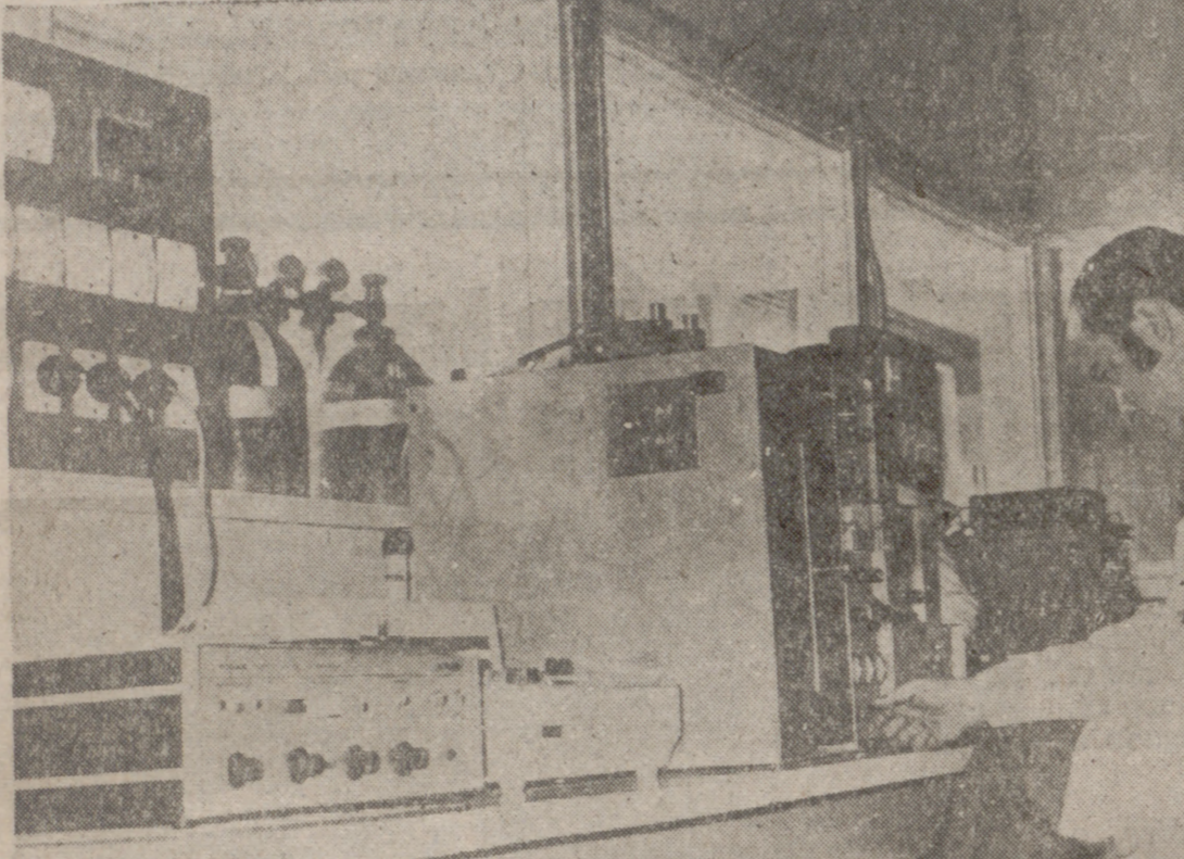
Determinación de los ácidos grasos del aceite de oliva por cromatografía gaseosa en el laboratorio de la C. A. T.
