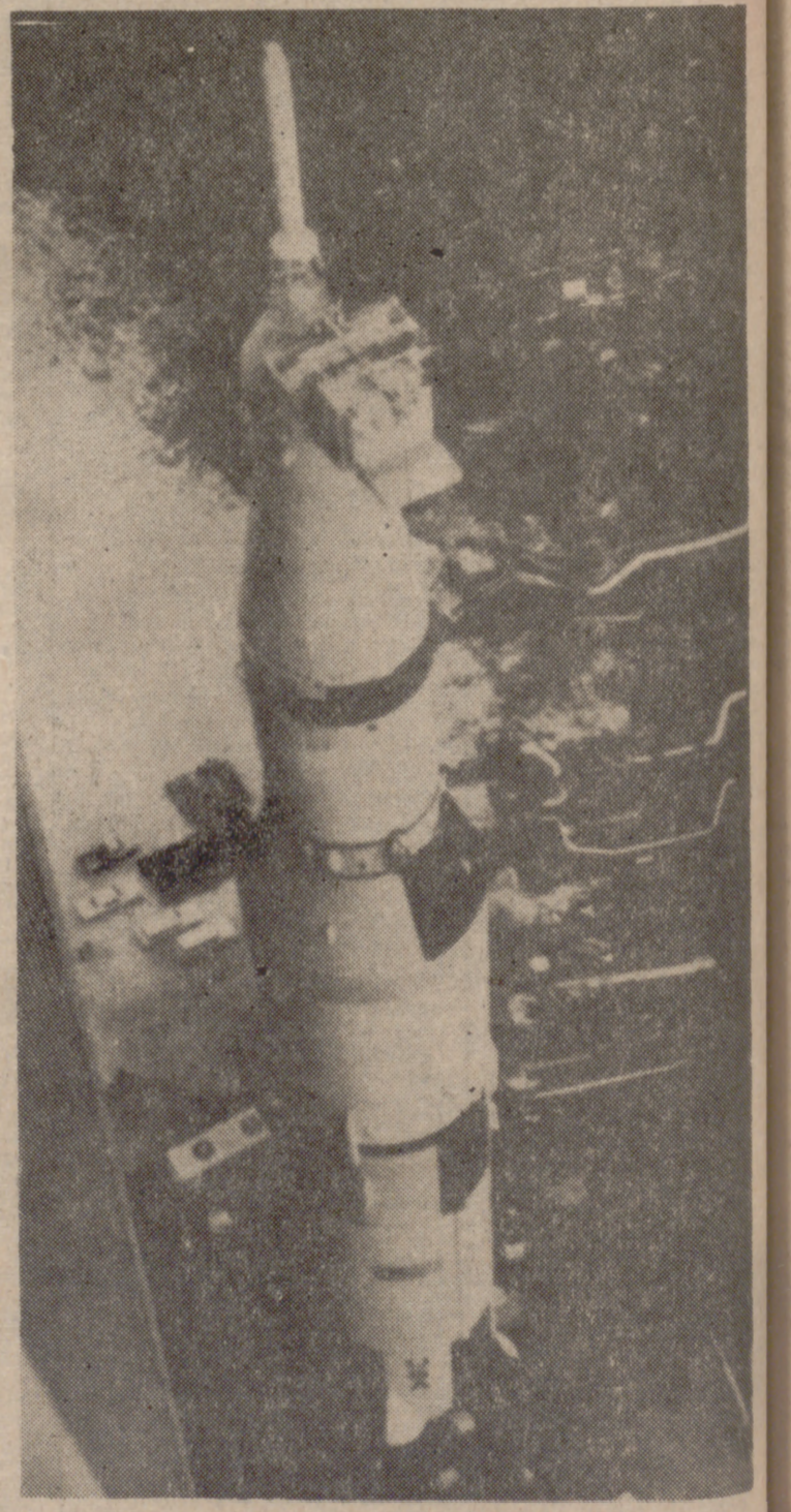
El gigantesco cohete «Saturno S-4 B», con el «Apolo XIV» montado sobre el extremo de su morro, en la pista de lanzamiento de Cabo Kennedy. En el extremo se distingue el cohete auxiliar de socorro de la cápsula.—(Foto PYRESA.)
