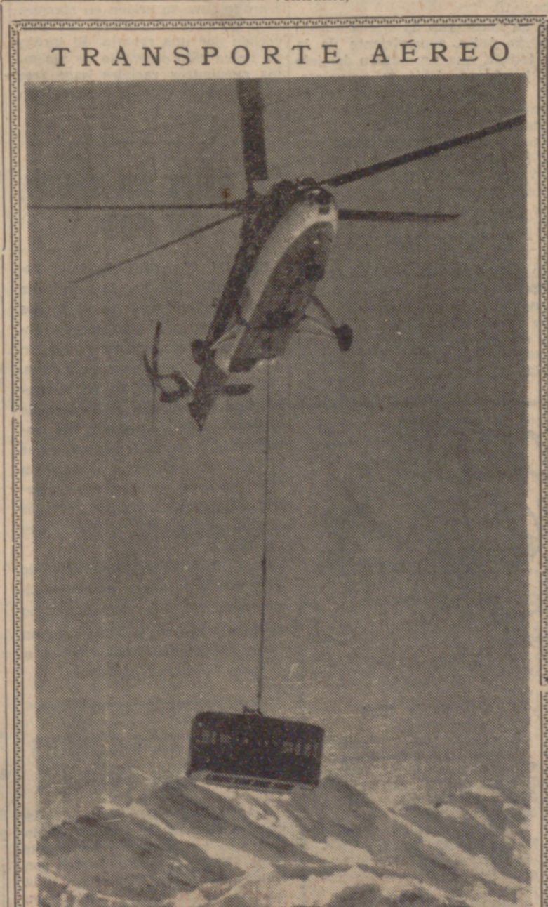
STECHELBERG.—Cien cabinas para pasajeros, con un peso de 1,2 toneladas, para el cable aéreo que se instala en los Alpes Berneses, han sido transportadas por helicópteros rusos "MI-6". En la foto, una de las cabinas citadas es transportada desde Stechelberg, a 667 metros, hasta Birg, a 2.677 metros. (Telefoto Cifra.)
