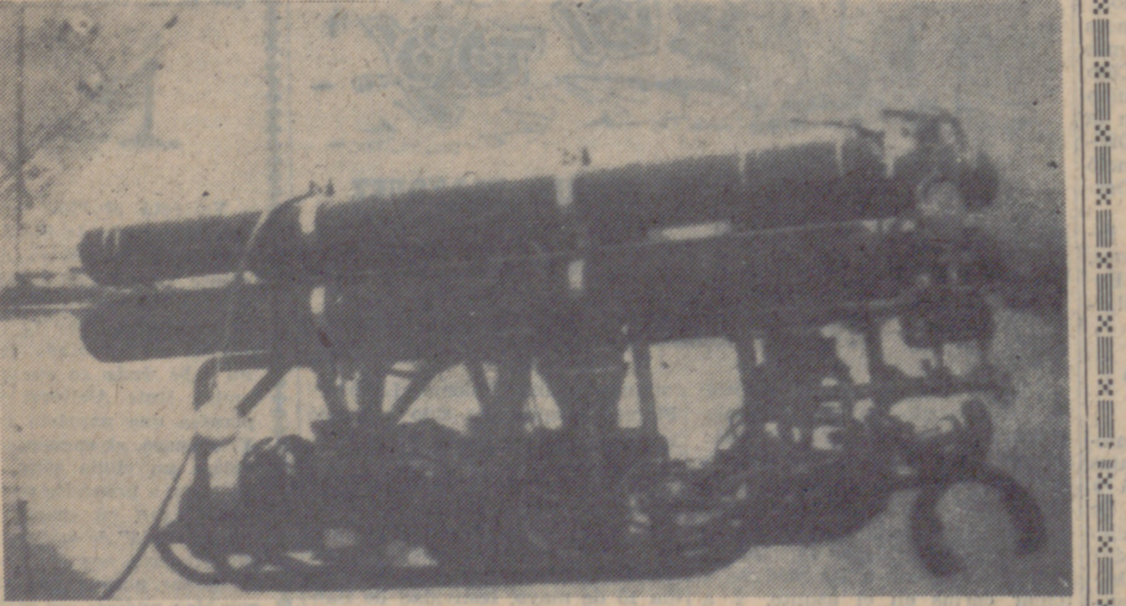
PALOMARES (Almería).—Este robot de la Armada de los Estados Unidos puede ser el aparato que extraiga esta semana la bomba desaparecida en el fondo del Mediterráneo, a una profundidad de 2.500 pies. Se llama "Curv" y está controlado por cables. El vehículo de investigación submarina tiene seis pies de alto, cinco de ancho y trece de largo. Está equipado con una cámara de televisión. Ha sido diseñado por la Naval Ordnance Test Station, en Pasadena (California).—(Telefoto Cifra.)
