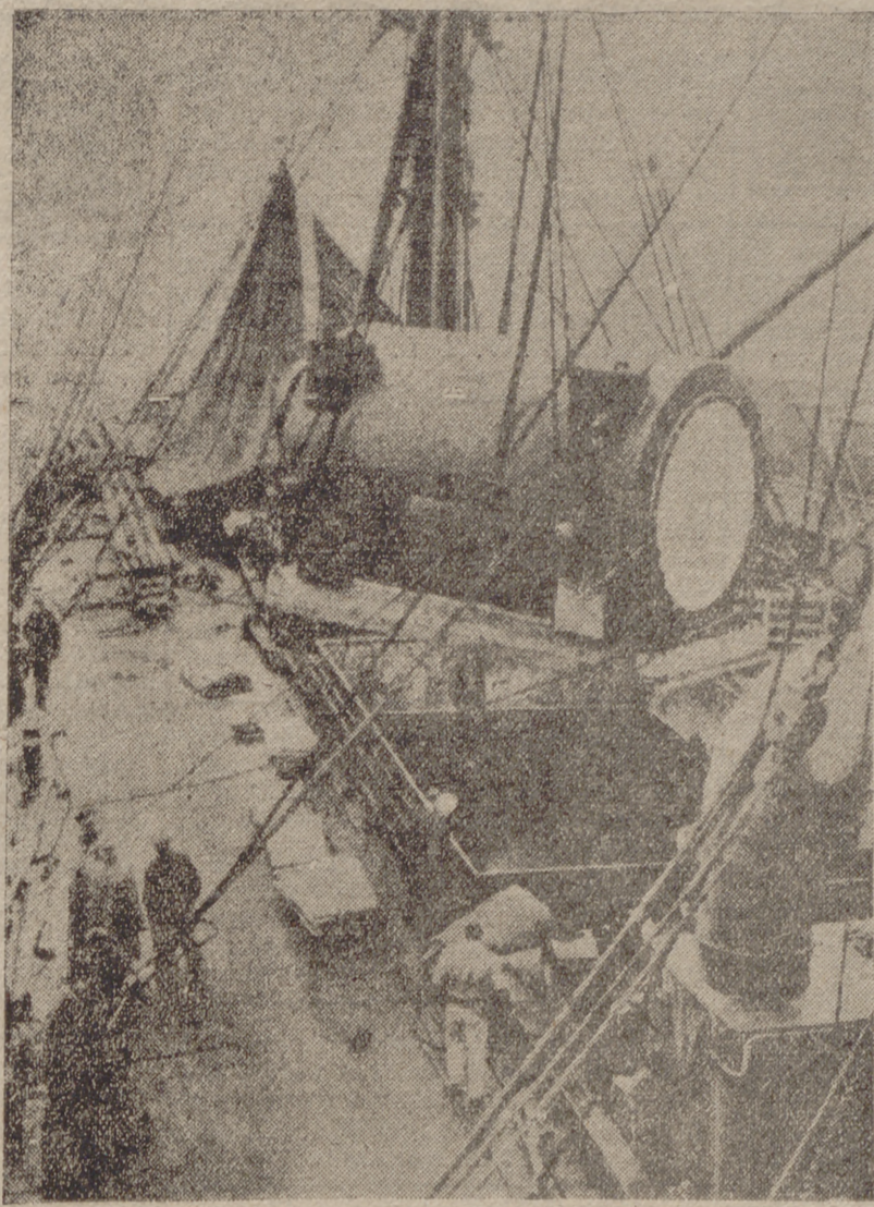
Un momento del embarque en Nueva York, a bordo del buque "Sete", de uno de los elementos de las tres turbinas de vapor con destino a la central eléctrica de Escambreras en Cartagena.
