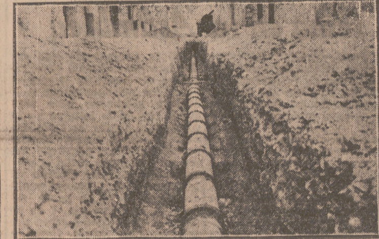
OBRAS DEL ALCANTARILLADO, EN CONSTRUCCION
