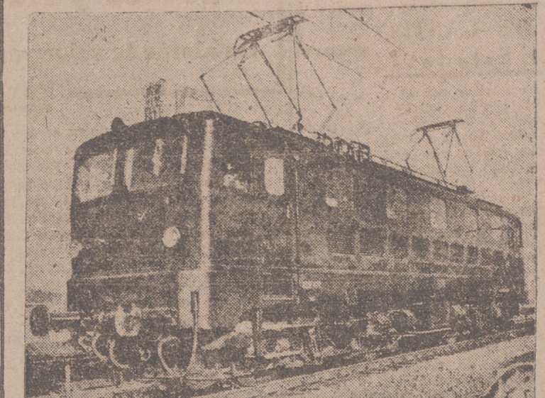
Nueva locomotora eléctrica B-B tipo 121
