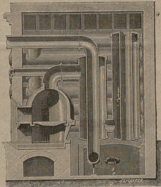
CALORIFÈRES A AIR CHAUD.
