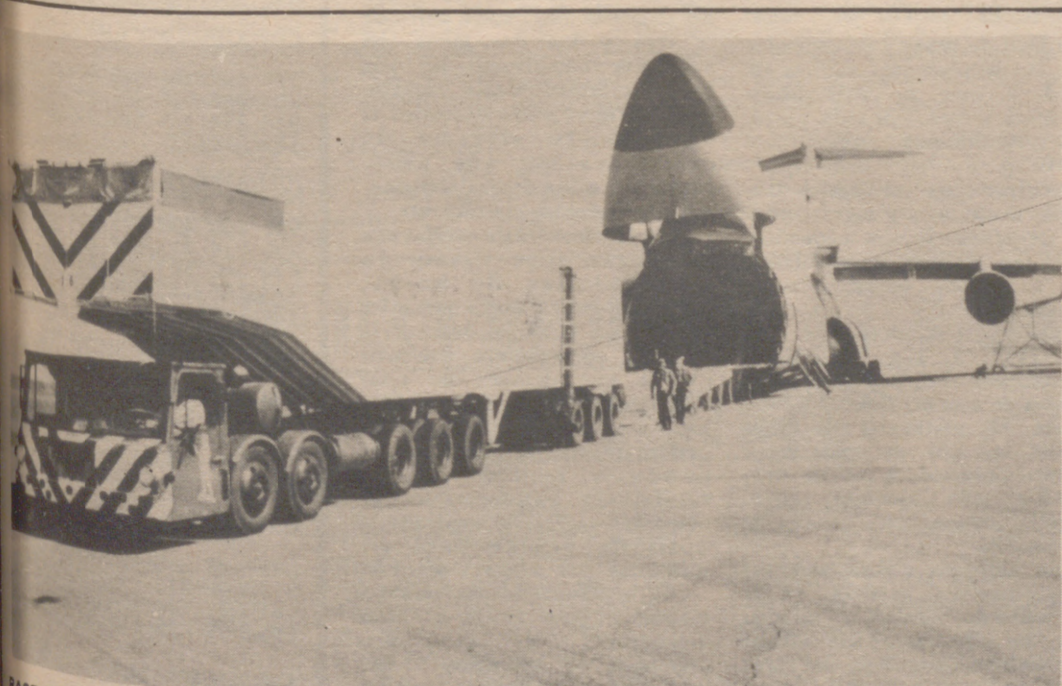
BASE AEREA DE HILL (Ogden, Utah, EE.UU).— El mayor avión transporte del mundo, un C-5 Galaxy, construido para las Fuerzas Aéreas norteamericanas por la "Lockheed", aparece en la foto cuando se va a introducir, a bordo, un tractor para el transporte de proyectiles "Minuteman III". Se asegura que el avión puede transportar hasta 390.000 kilos de carga
