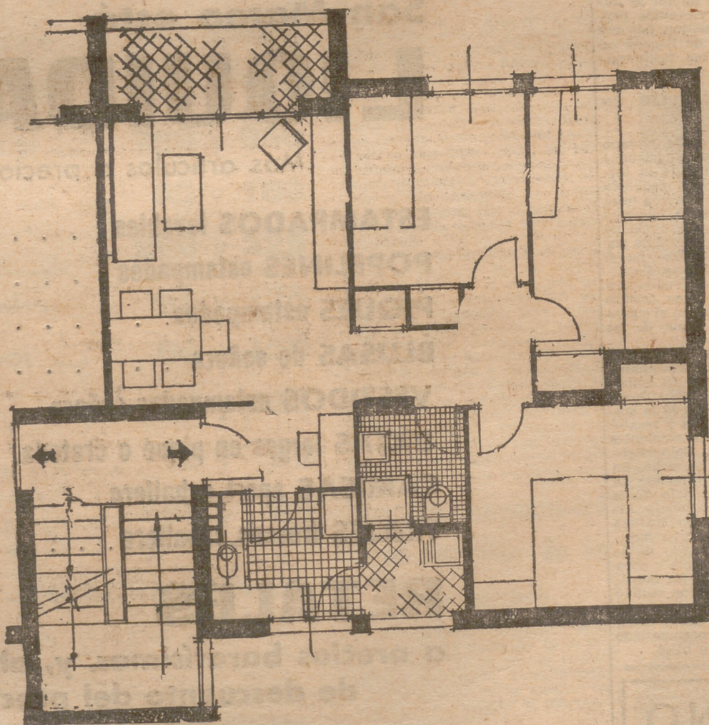
PISO TIPO «A»
