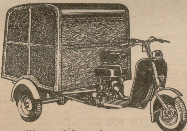
"Motofurgón" con caja cerrada y acceso posterior
