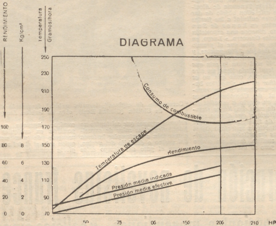
Diagrama indicador del consumo de combustible, temperatura de escape, presiones y rendimiento de un motor Diesel T. E. B. de 200 HP, a 460 revoluciones por minuto, y cuatro cilindros. Puede observarse cómo el consumo de combustible es muy reducido, aun en casos de poca carga, con una temperatura de escape baja, siendo las presiones muy moderadas y un alto rendimiento del motor.
