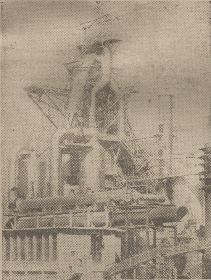
El horno alto número 1, la depuradora de gas, de la gigantesca factoria siderúrgica de Avilés
