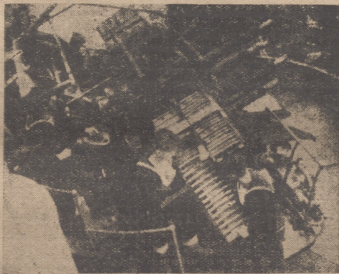
Para combatir a los "Stukas" los ingleses han dotado a la mayor parte de sus unidades navales de este tipo de cañón múltiple llamado "pom-pom". Según los técnicos británicos, es la más eficaz arma anti-aérea. Por sus seis bocas el "pom-pom" puede hacer eléctricamente centenares de disparos al minuto.
